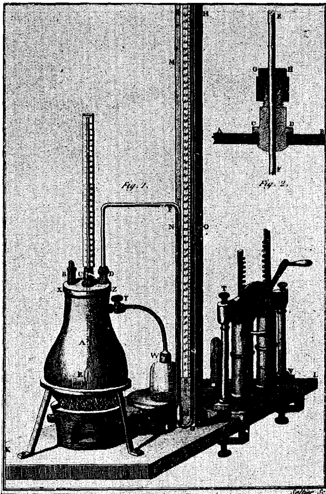
Dibujo de la Mémoire sur la force expansive de la vapeur de l'eau de don Agustín de Béthencourt, impresa en París (Fotografía comunicada por don Antonio Ruiz Álvarez)
