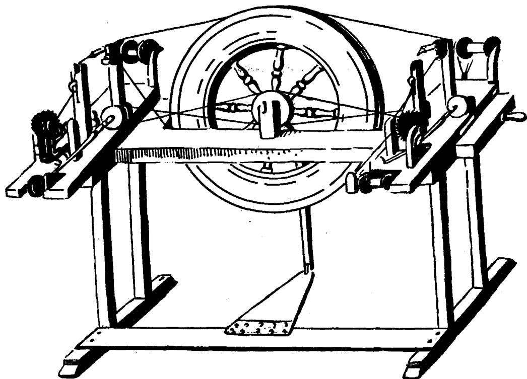
Máquina epicilíndrica para hilar seda, inventada por don Agustín de Béthencourt y Molina, en Santa Cruz de Tenerife, 1778
